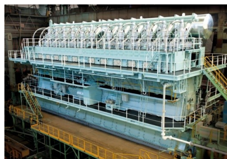
12RT_flex96C エンジン
