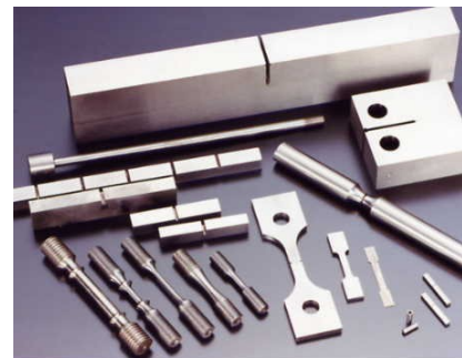
各種金属材料試験片
